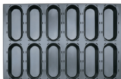
SN9051 12连长条型模(800系列不沾) SN9054 12连长条型模(1000系列不沾) 规格: 600x400x42mm
