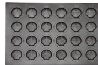
SN9044 24连深贝壳模(800系列不沾) 600x400x24mm
