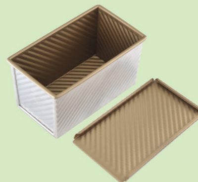
SN2089 1.0mm铝合金 450g波纹土司盒(1000系列不沾) 内径196x106x110mm
