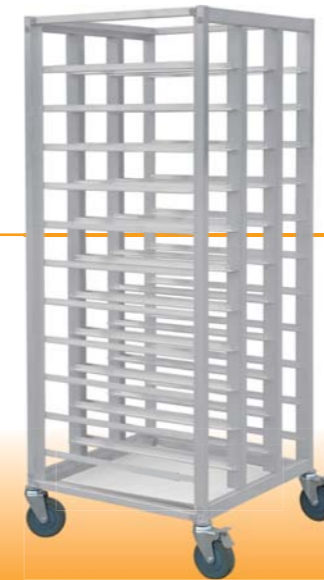
SN1993 层高:126mm 适合6"和8"蛋糕模 11层组合式蛋糕模冷却车(阳极) 809x750x1695
