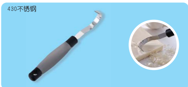
SN4063 巧克力刮刀 总长203刃长72
