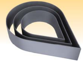
SN3905 6" 水滴型圈 (硬膜) 152x108x50 SN3906 8" 水滴型圈 (硬膜) 203x144x50 SN3907 10" 水滴型圈 (硬膜) 254x179x55
