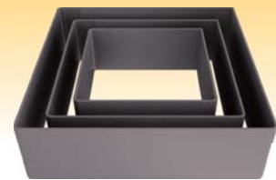
SN3880 6" 四方圈 (硬膜) 108x108x50 SN3881 8" 四方圈 (硬膜) 144x144x50 SN3882 10" 四方圈 (硬膜) 180x180x55
