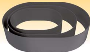
SN3870 6" 橢圓圈 (硬膜) 152x110x50 SN3871 8" 橢圓圈 (硬膜) 203x145x50 SN3872 10" 橢圓圈 (硬膜) 254x180x55
